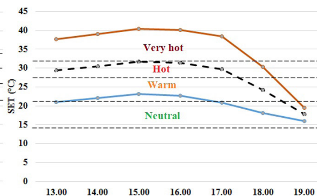
نمودار ۸. حداکثر، حداقل و میانگین SET* سناریوی A-3 بین ساعت ۱۳:۰۰ تا ۱۹:۰۰ روز ۲۱ ژوئن در مقایسه با تنش حرارتی بین‌المللی (سمت چپ) و مقیاس اصلاح‌شده برای تهران (راست)
