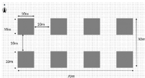
شکل ۲: ساختار بلوکی شرقی
