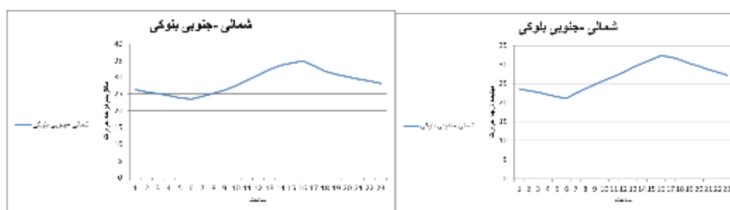
نمودار ۲: تاثیر نحوه استقرار ساختمان بلندبه صورت بلوکی در جهت گیری شمالی-جنوبی بر ماکزیمم و مینیمم درجه حرارت
